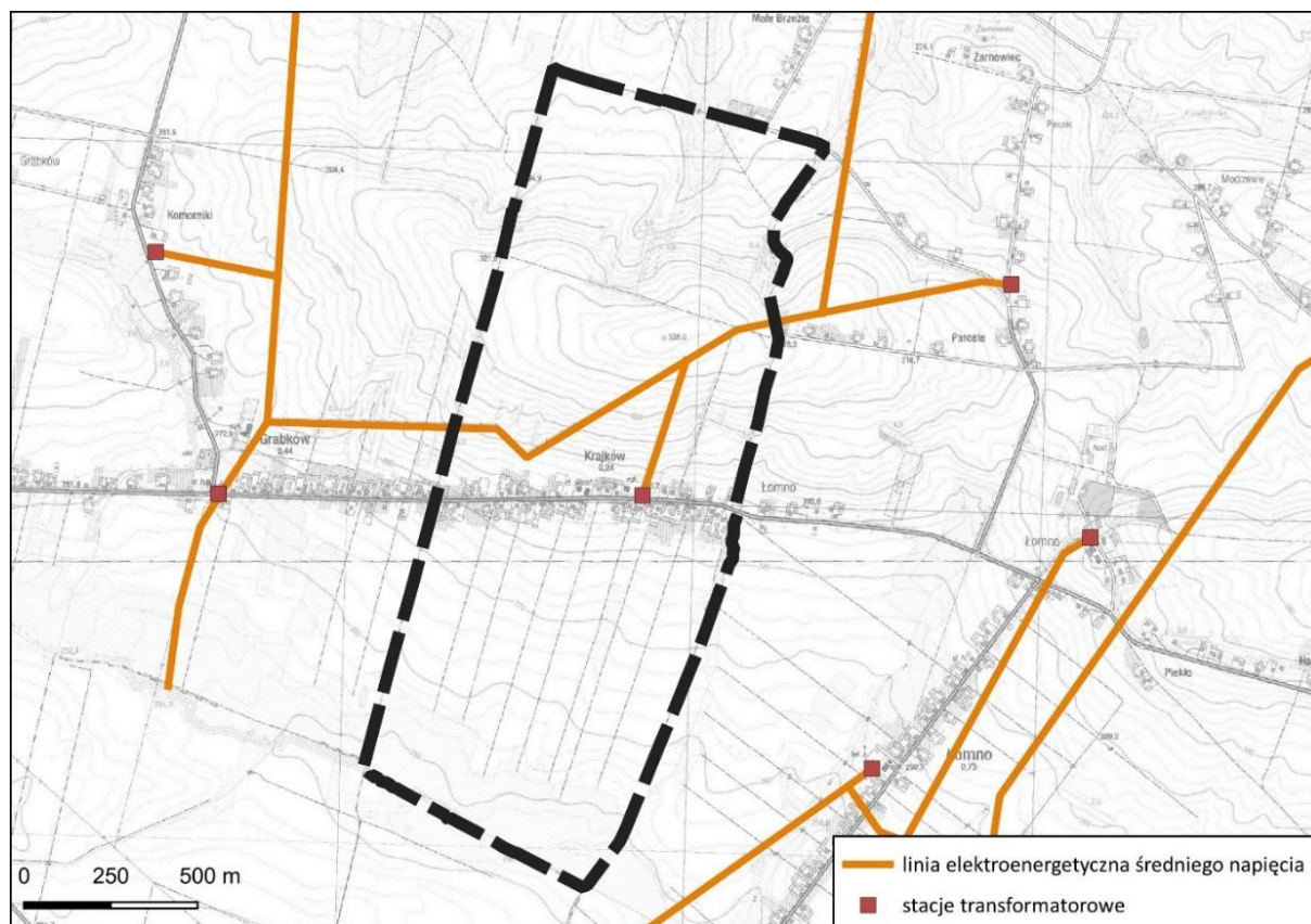
Rysunek 10. Przebieg linii elektroenergetycznych na terenie opracowania
